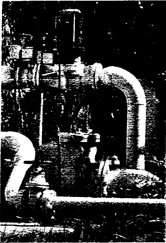
17.เครื่องเพิ่มแรงดันน้ำประปาปลายทาง (In line Pump) ขนาดส่งน้ำได้ 60 ลบ.ม./ชม. ที่ส่งสูงได้ 40 เมตร ขับเคลื่อนด้วยมอเตอร์ไฟฟ้า ขนาด 20 Hp(15 KW) พร้อมอุปกรณ์ พร้อมตู้ควบคุมเครื่อง เลขที่พัสด 055-43-0012
